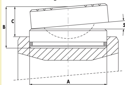
bewegliches Druckstück
